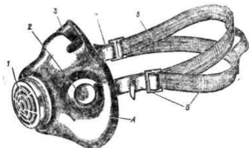
Рис. 19. Респиратор Р-2:
