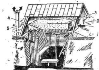
Рис. 8. Оборудование первого этажа (а), подвального помещения (б), погреба (в) под противорадиационное укрытие.
