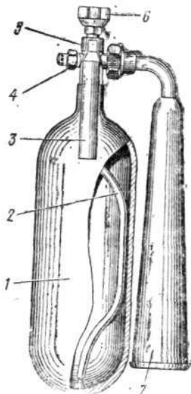
Рис. 30. Устройство углекислотного огнетушителя;
