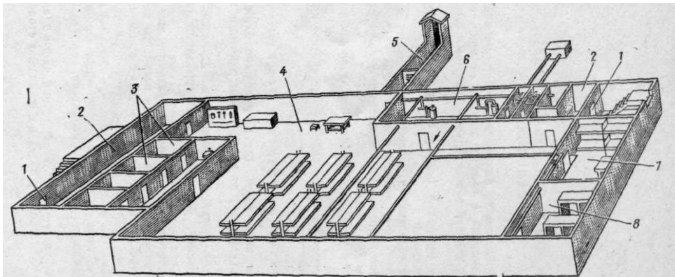
Рис. 6. План убежища:
