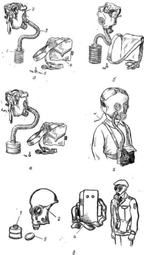
Рис. 14. Детские фильтрующие противогазы: а — противогаз ДП-6м; б — противогаз ДП-6; а — противогаз ПДФ-7; г — противогаз ПДФ-Д; д — противогаз ПДФ-Ш (со шлемом-маской); 1 — фильтрующе-поглощающая коробка; 2 — лицевая часть (у противогаза ПДФ-Ш — шлем-маска, у остальных противогазов — маска); 3 — соединительная трубка; 4 — сумка для противогаза; 5 — специальный «карандаш»; 6 — незапотевающие пленки
