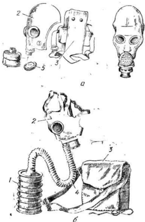
Рис. 12. Фильтрующие противогазы:
